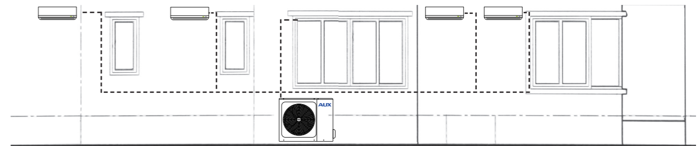
Pięć jednostek wewnętrznych w systemie multi split
